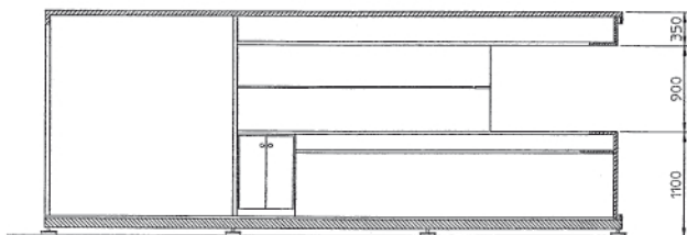
L=6 m. SECCIÓN A-A' / SECTION A-A'
