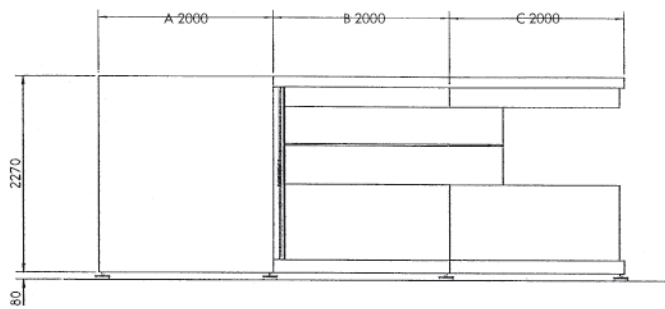
L=6 m. ALZADO FRONTAL ABIERTO / SIDE VIEW OPEN
