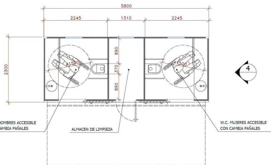
1 PLANTA DISTRIBUCION
